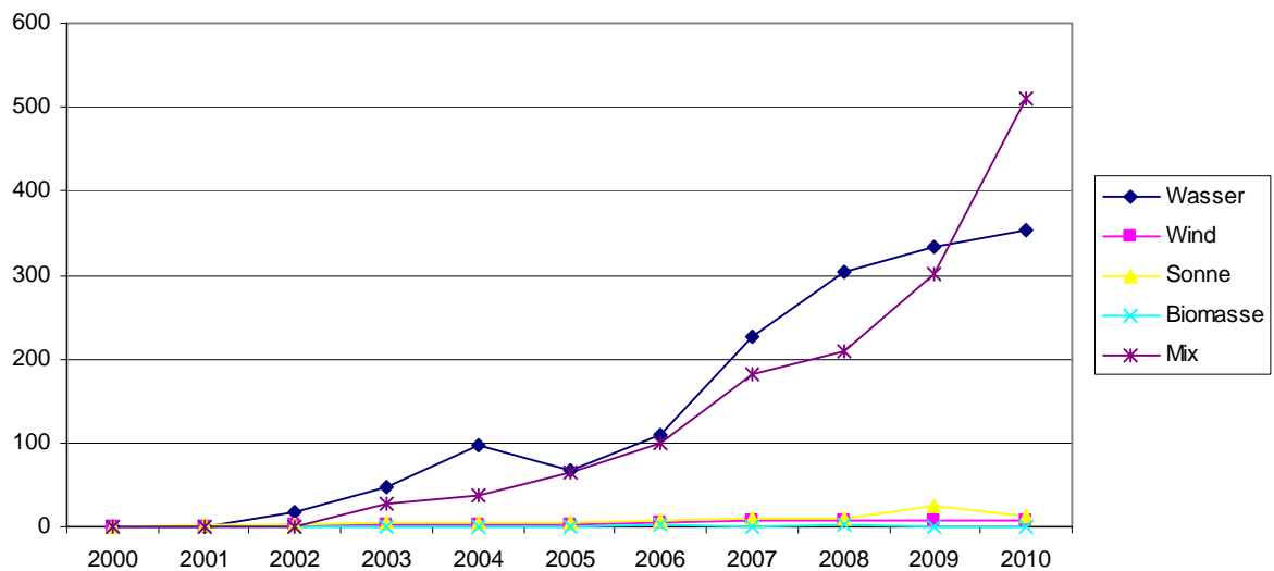
Grafik 2: Verkaufszahlen naturemade star 2001 - 2010 (GWh) Aufgeschlüsselt nach Energiesystemen
